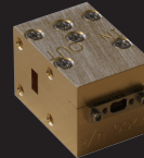
LNF-LNR28_52WA (28GHz-52GHz/waveguide)
