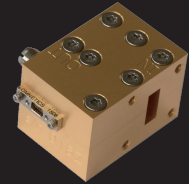
LNF-LNR16_28WA (16-28GHz/waveguide)
